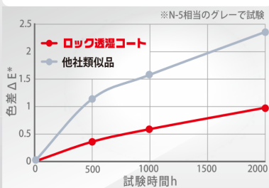
促進耐候性 (キセノンウェザーメータ)
